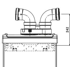
CONDOTTI SDOPPIATI Ø 80-80 CON ADATTATORE
