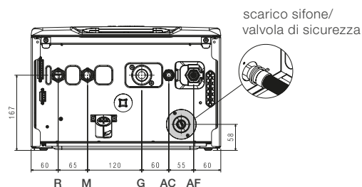
VISTA DAL BASSO (SENZA COPERTURA)
